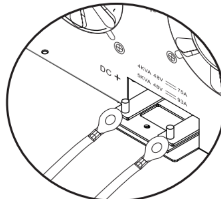
4~5кВА
