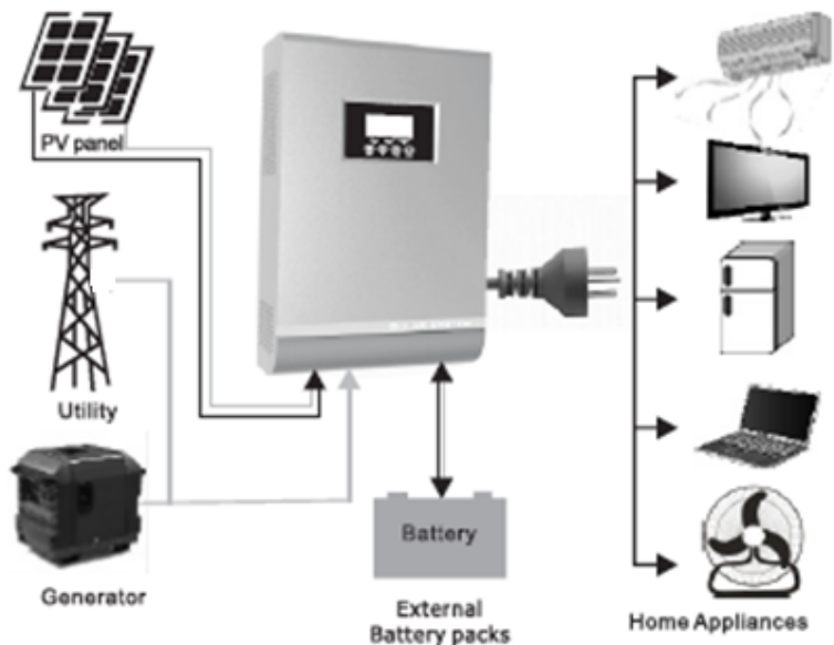
Рис. 1 Гибридная электрическая система
