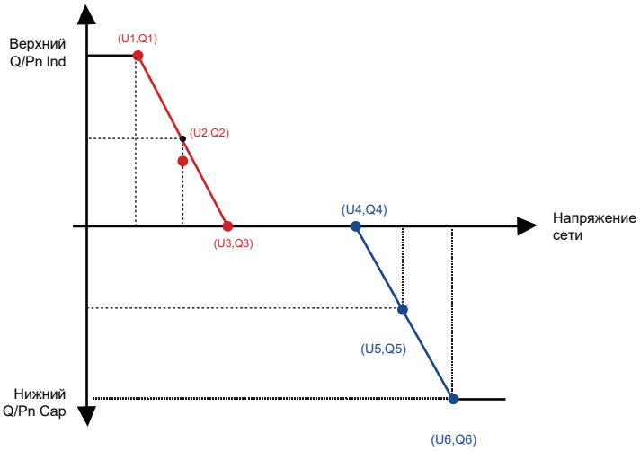
Рис. 8.26 Кривая регулирования реактивной мощности в режиме Q (U)
