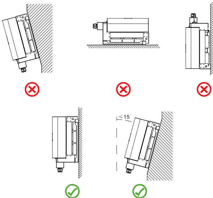
Рис. 4.2 Угол установки
