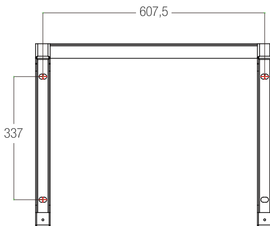
Рис. 4.3 Зазор при установке
