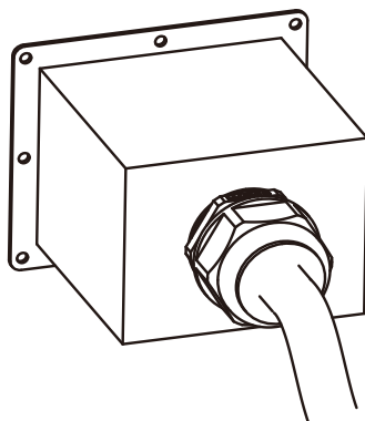
Рис. 5.11 Фиксация распределительной коробки перем. тока
