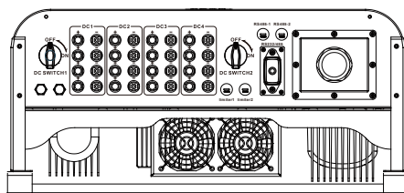
Рис. 1.2 Вид сзади
