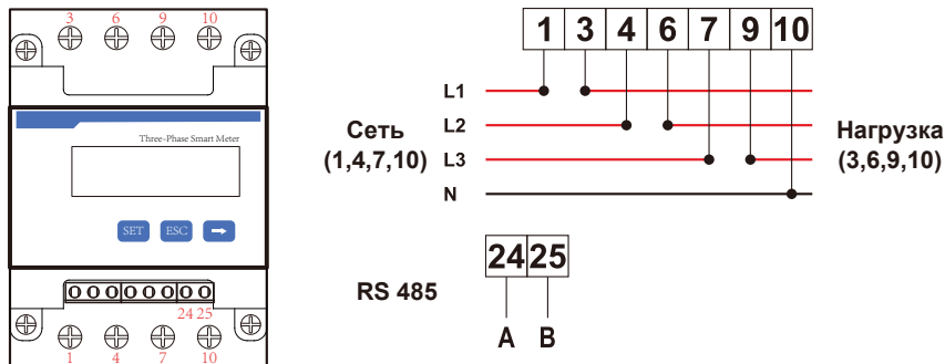
Рис. 7.5 Счетчик CHNT
