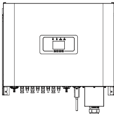
Рис. 1.1 Вид спереди
