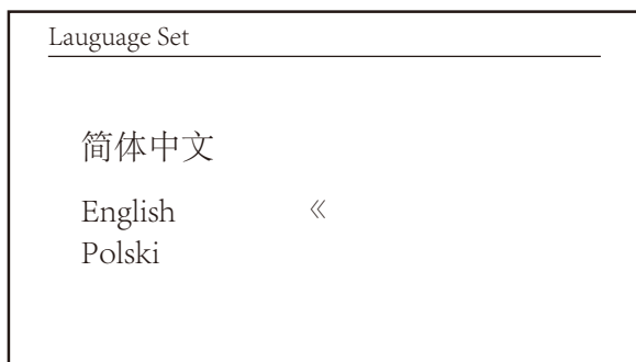
Рис. 8.20 Настройки языка
