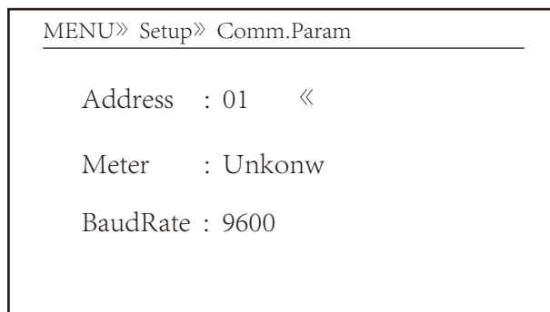
Рис. 8.32 Параметры связи
