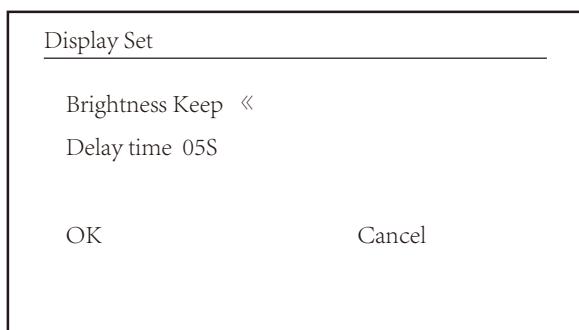
Рис. 8.21 Настройки отображения
