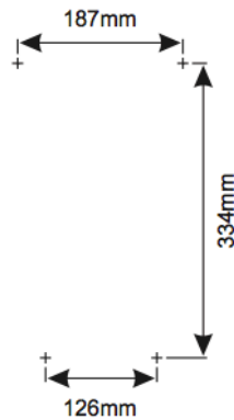
Расположение крепежных отверстий
