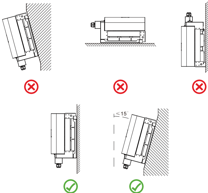
Рис. 4.2 Угол установки
